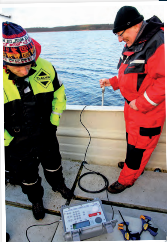
Fra den første "lyttetur" i forbindelse med vandringsprojektet. Det foregår med håndholdt antenne i Roskilde Fjord.
